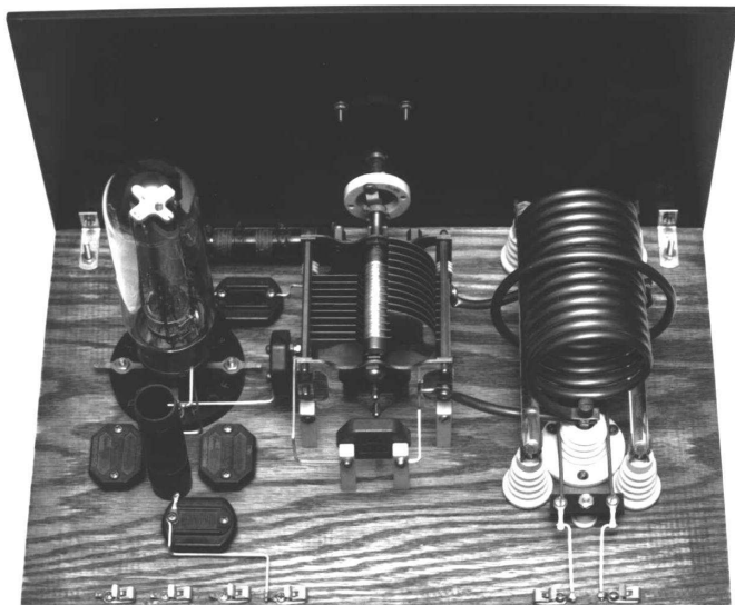
Oscilatorul Armstrong
