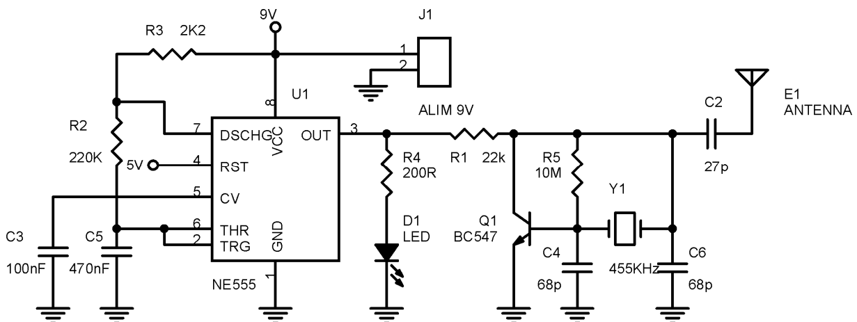
Schema electrică
