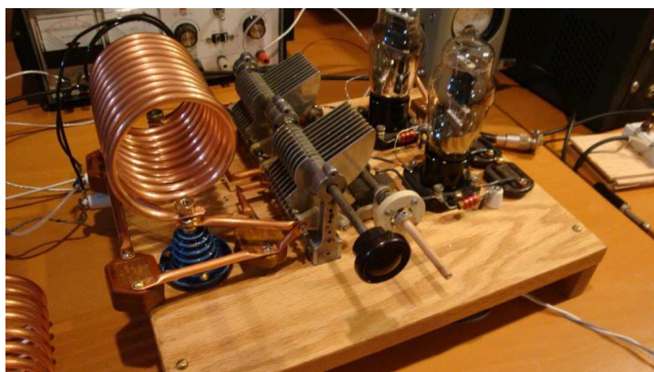
Emițătorul Colpitts
