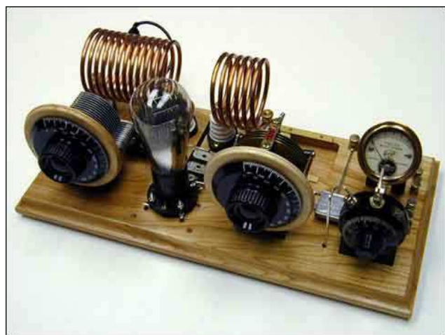
Oscilatorul Hartley
